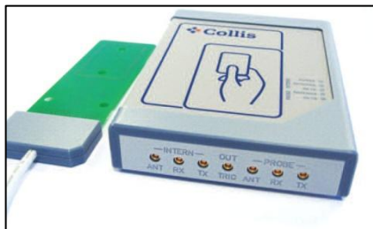
Устройство SmartWave Box компании Collis для имитации бесконтактных карт
